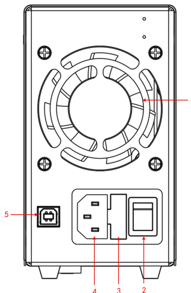
Abbildung 2-2 Übersicht der Rückseite
