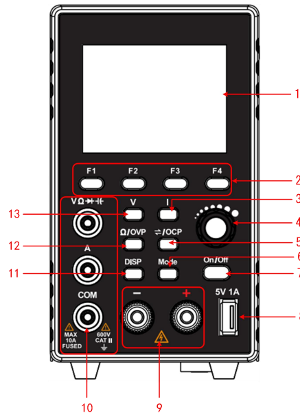
Abbildung 2- 1 Übersicht der Vorderseite
